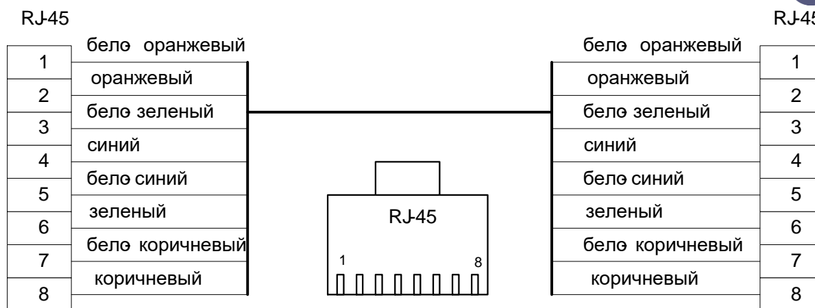
Рисунок 7.4 - Разделка кабеля.
