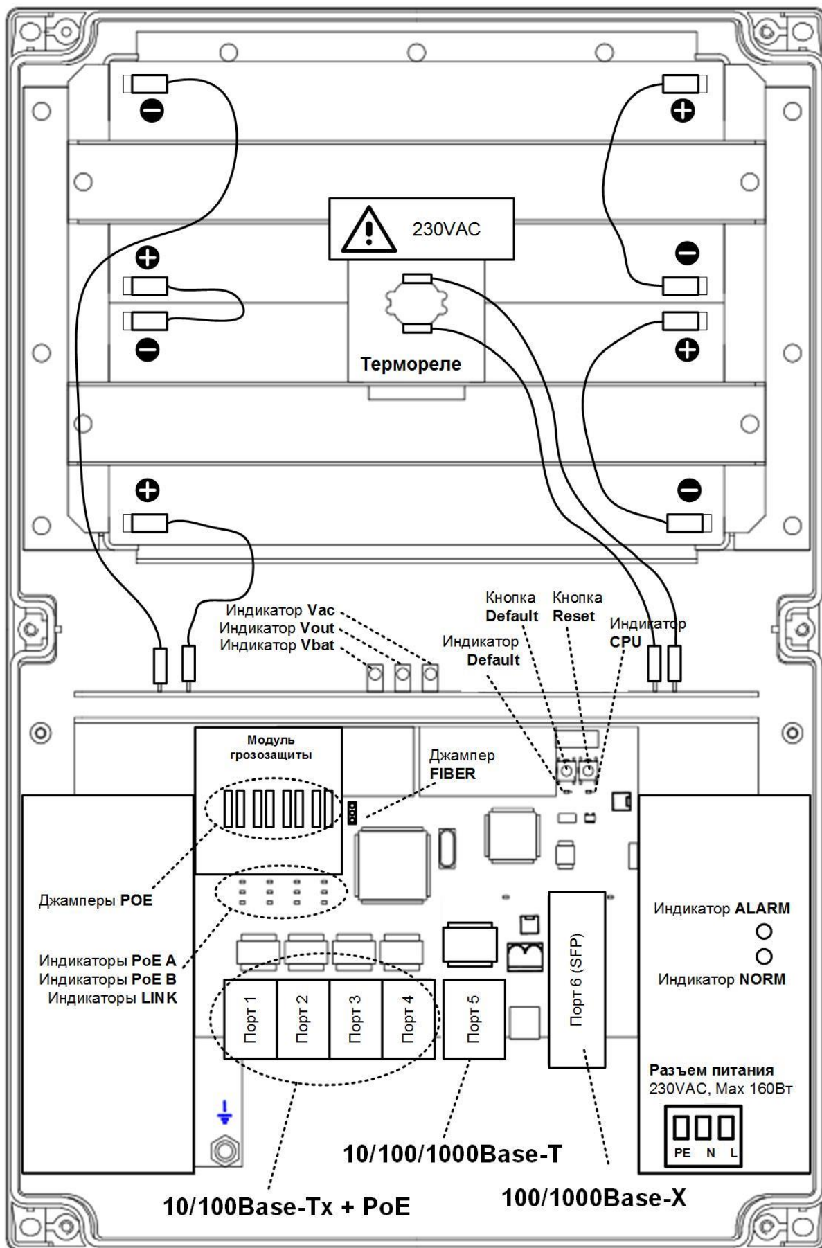
Рисунок 3.2.2 - Расположение элементов PSW -1G4F-UPS
