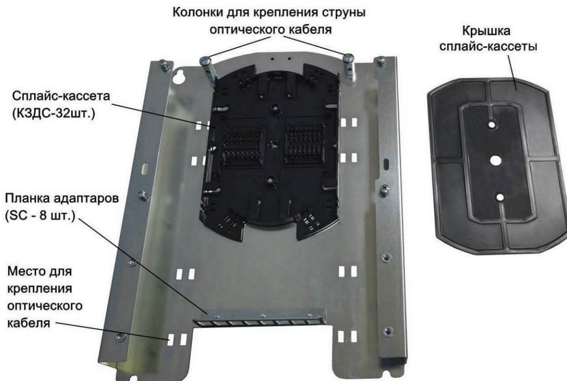
Рисунок 3.3 - Оптический кросс
