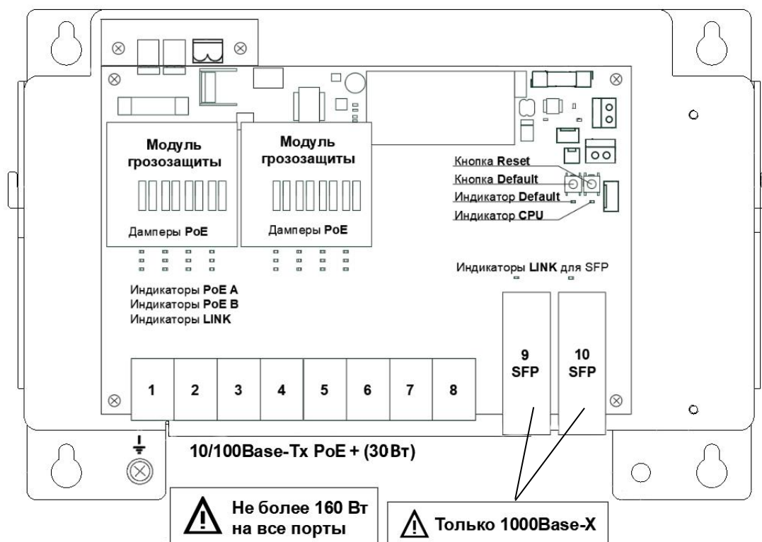
Рисунок 3.4.2 - Расположение элементов PSW-2G8F+Box
