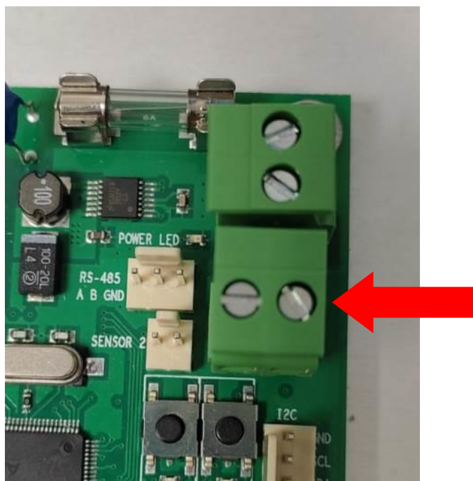
Рисунок 3.5 - сухой контакт.
