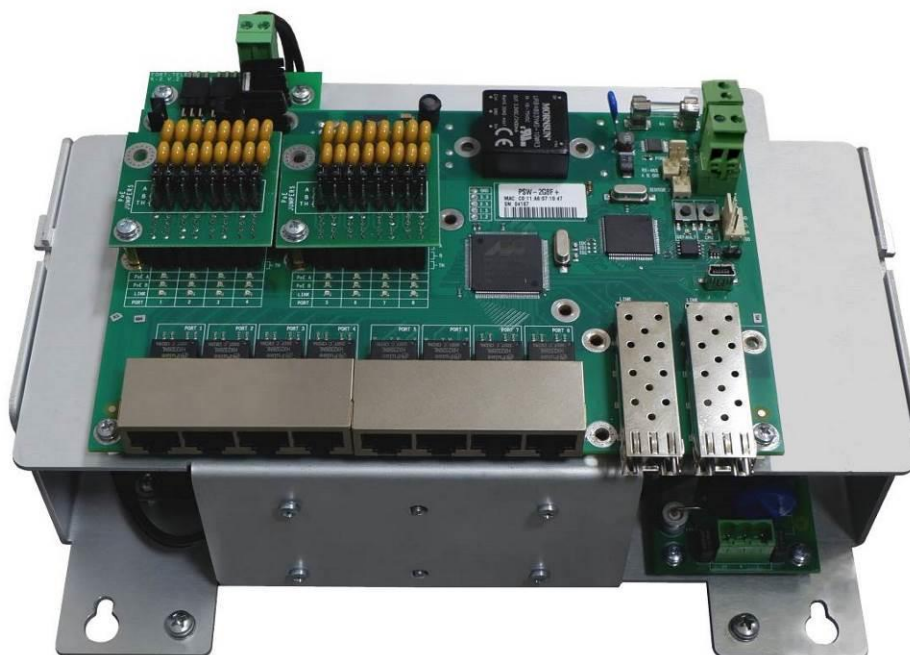
Рисунок 3.4.1 - Плата коммутатора и блоков питания
